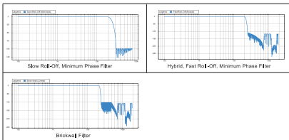
数字滤波器的频率响应曲线
